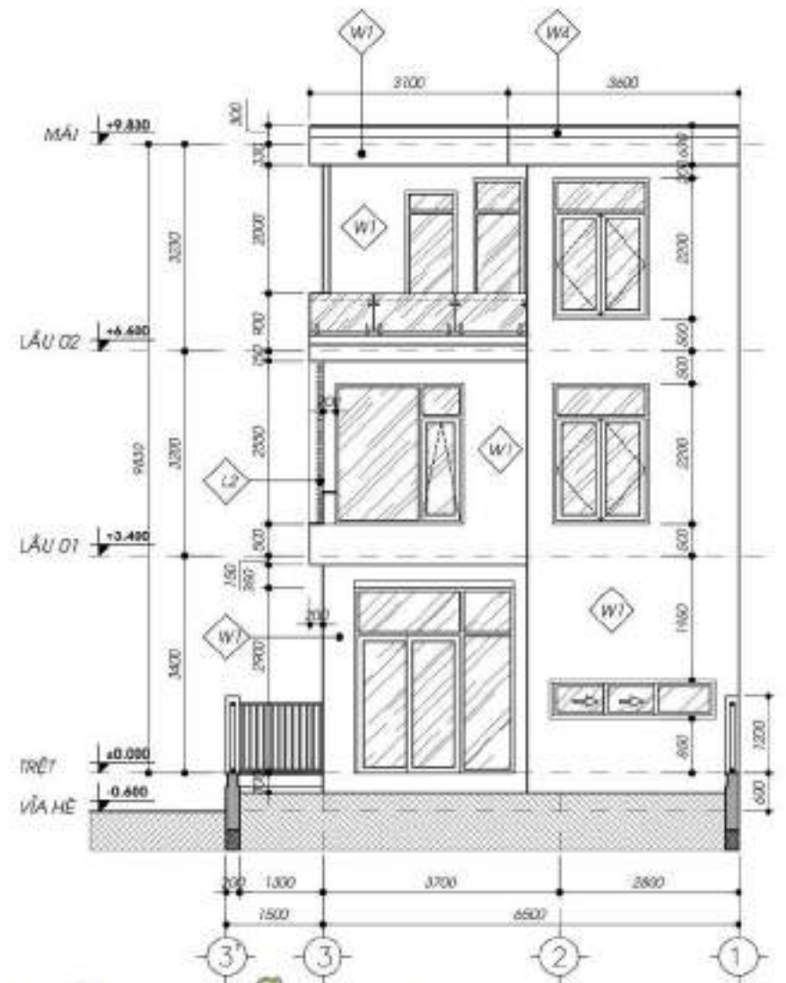
MẶT BẰNG TRỰC ĐỨNG - MẪU M3
